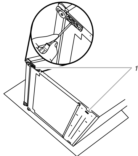
1. Vis Phillips
