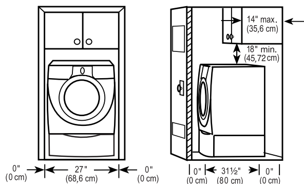
1 1. Encastrement 2. Vue latérale - placard ou endroit exigü
