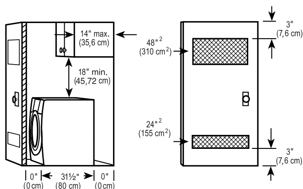
1 1. Vue latérale - placard ou endroit exigü 2. Porte de placard avec orifices d'entrée d'air
