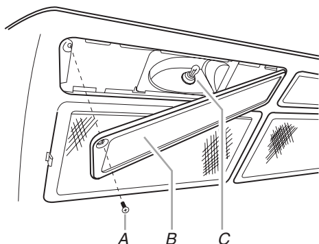
A. Vis de montage B. Couvercle de l'ampoule C. Ampoule halogène
