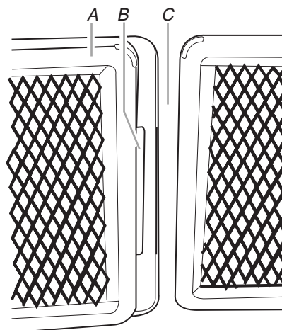
A. Cadre du filtre B. Onglet large C. Fond du four à micro-ondes
