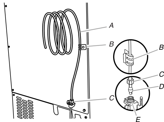
A. Tubería de cobre de 1/4"
