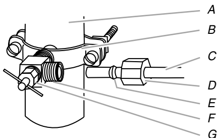
A. Canalisation d'eau froide B. Bride de tuyau C. Tube en cuivre D. Écrou de compression E. Bague de compression F. Robinet d'arrêt
