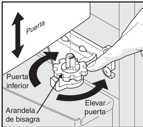
Levantar/bajar puerta
