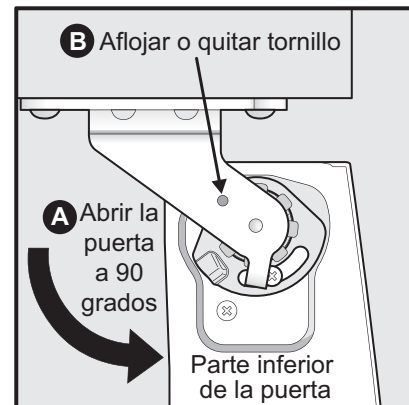
Aflojar/quitar tornillo
